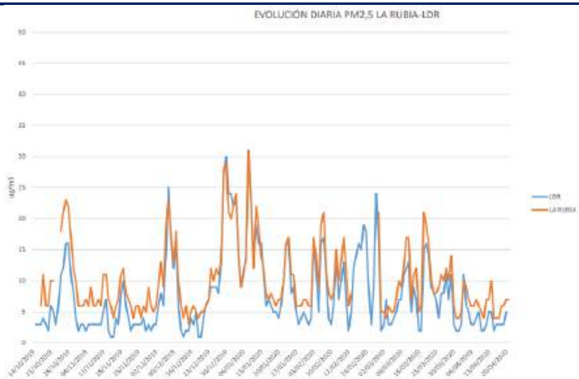
Gráfico 3: Evolución de las medias diarias de PM2,5 (µg/m3) en la estación de La Rubia y LDR.
