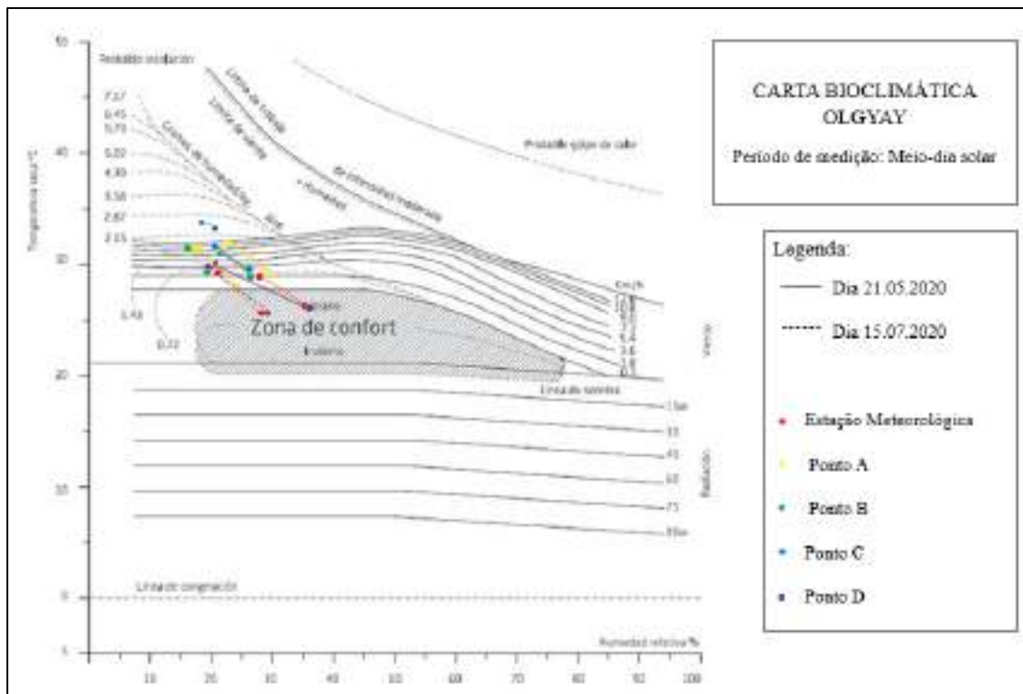
Fig. 52 - Carta bioclimática de Olgyay para los cuatro puntos de medición en el periodo de mediodía solar para el 21 de mayo y el 15 de julio de 2020.
