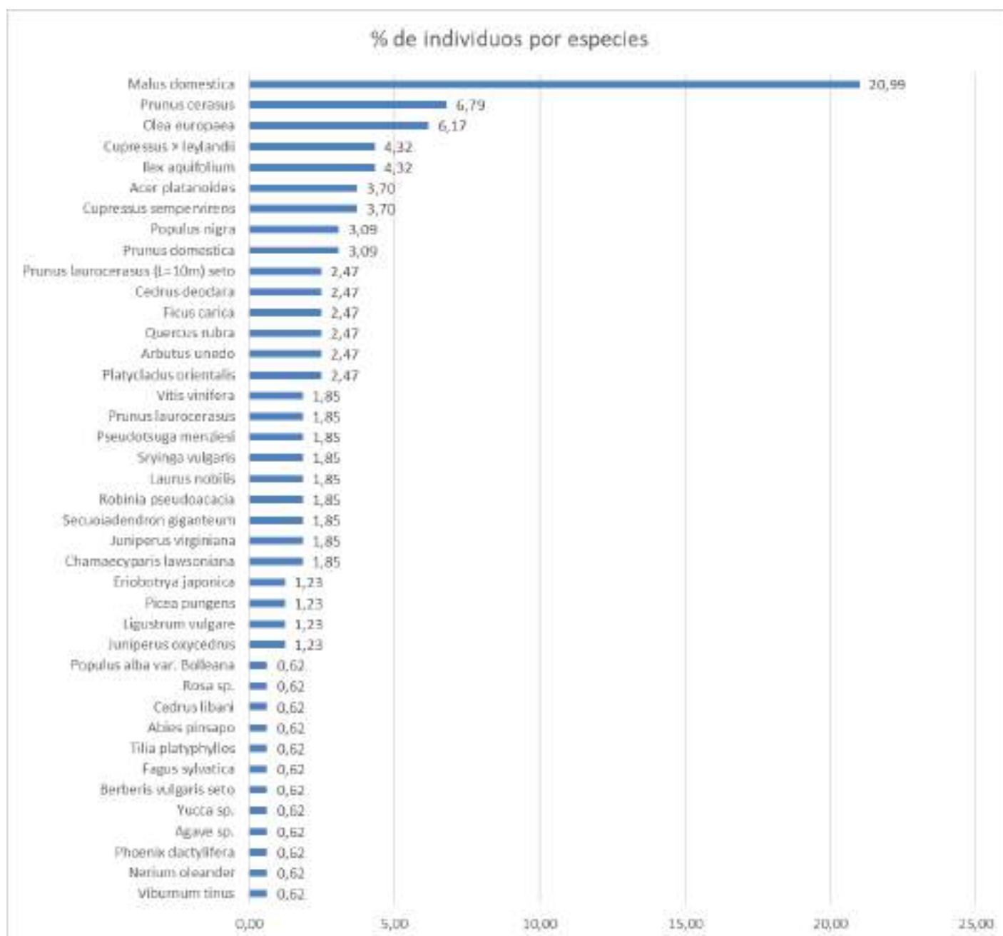
Fig. 33: Porcentaje de individuos por especie. Árboles y arbustos en privado. Fuente: elaboración propia
