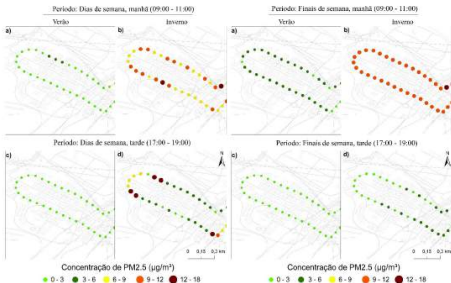
Fig. 43- Concentraciones de PM 2,5 en las calles del Polígono Industrial de Cantarias. A la izquierda están los valores de los días laborales, mientras que a la derecha están los valores del fin de semana. Ambas cifras están divididas por estación y periodo de muestreo, para cubrir las diferentes condiciones atmosféricas locales en las distintas estaciones.
