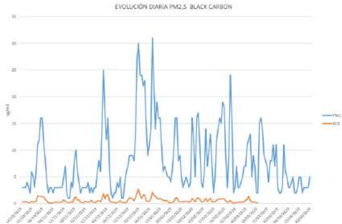
Gráfico 9: Evolución de los valores medios diarios de PM2,5 con longitud de onda del canal bc9 (µg/m3) en la estación LDR.
