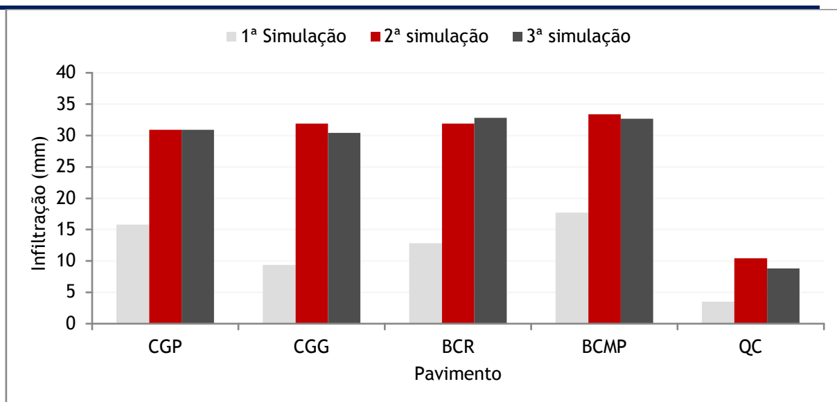
Fig. 61 - Cantidad de agua de infiltración para pavimentos contruidos con cubos de granito pequenos (CGP), cubos de granito grandes (CGG), bloques de cemento rectangulares (BCR), bloques de cemento tipo "mapa de Portugal" y cuadrados de cemento (QC)
