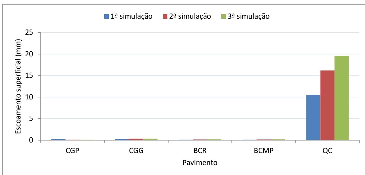
Fig. 62 - Cantidad de agua de escorrentía en pavimentos contruidos con cubos de granito pequenos (CGP), cubos de granito grandes (CGG), bloques de cemento rectangulares (BCR), bloques de cemento del tipo "Mapa de Portugal" y cuadrados de cemento (QC)
